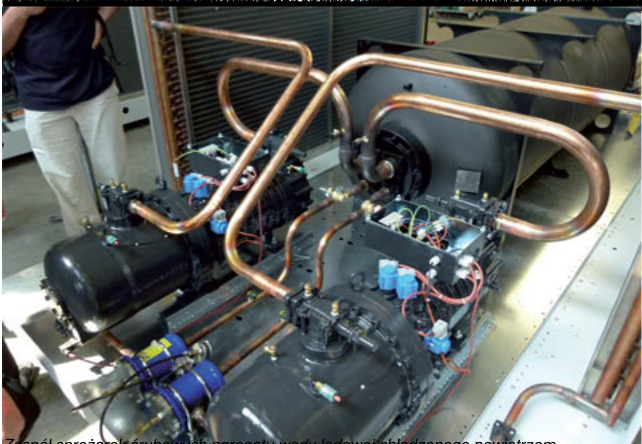
Zespół sprężarek śrubowych agregatu wody lodowej chłodzonego powietrzem
